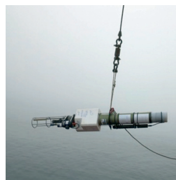
Déploiement d'un Pro-Ice (équipé de capteurs BGC) en Baie de Baffin (site BB2, juillet 2017, Navire Amundsen, mission AN1702). © Claudie Marec
