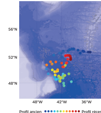
Figure 2b: Trajectoire du flotteur 6901758 déployé dans la zone de Fracture Charlie Gibbs.
