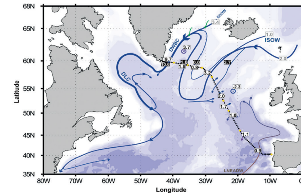
Figure 2a: Carte des courants moyens profonds (Daniault et al. 2016).
