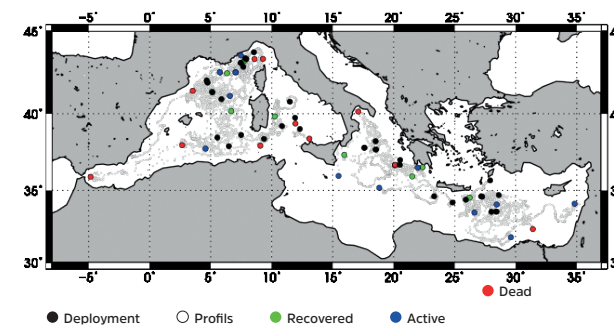
Position des profils BGC-Argo du réseau NAOS en Méditerranée.
