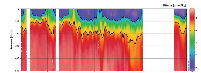
Évolution de la concentration en nitrates obtenue à partir des flotteurs BGC NAOS.
